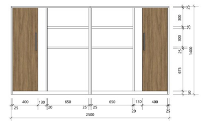
组合办公套装(柜) 正立面图1: 20
