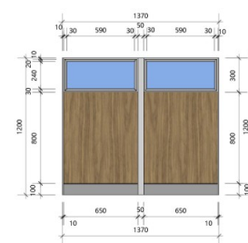
组合办公套装(隔断) 侧立面图1: 20
