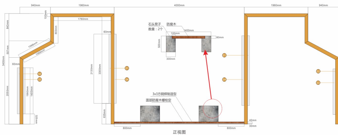
正视图
